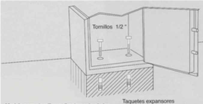
Modelo para atornillarse directamente al piso
